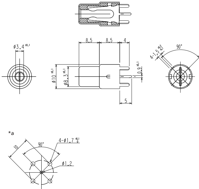
*a Leiterplattenlayout
