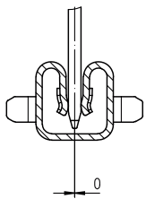
typische Kontaktierung
