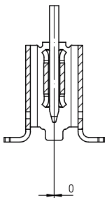
typische Kontaktierung
