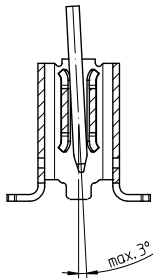
zulässige Neigung
