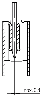
zulässiger seitlicher Versatz
