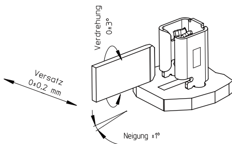
zulässige kombinierte Toleranzen
