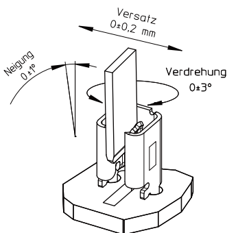
zulässige kombinierte Toleranzen
