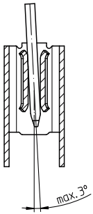
zulässige Neigung
