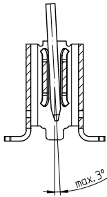
permissible tilt
