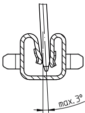
permissible tilt
