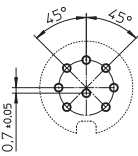
08-a KFR 81
