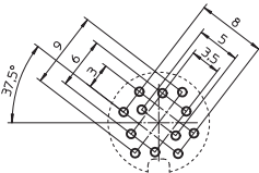
12-a KFR 120
